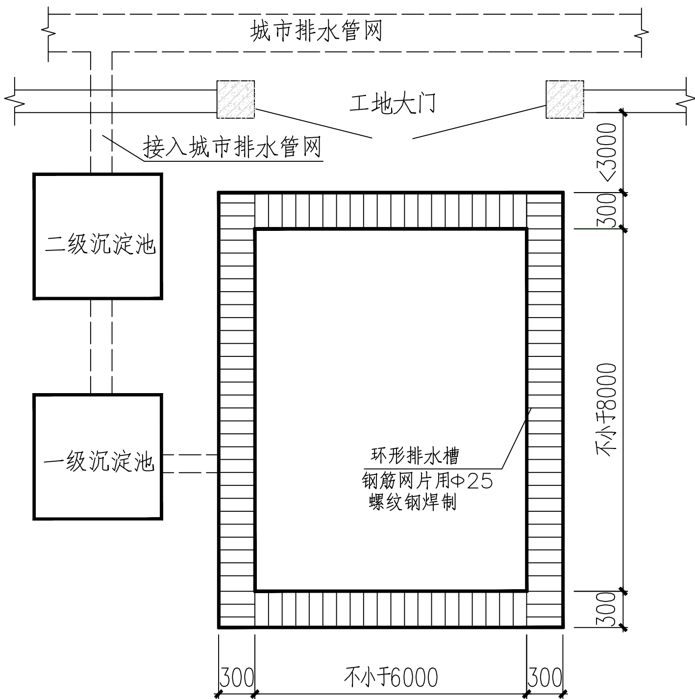
工地冲洗平台示意图
